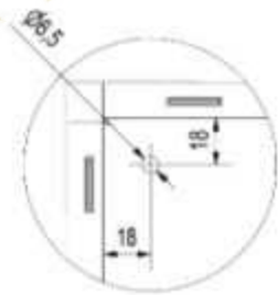
Otwór montażowy mierzony od krawędzi komory spalania
